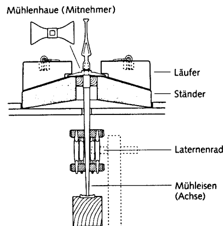
Schnell laufendes Mahlwerk mit Getriebeteilen nach dem Fund von Zugmantel, Taunus (2. H. 2. Jh. n. Chr.).
